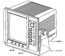
登録 01170454 船舶レーダ用指示機
