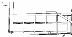
G2-2914 登録1122650号 貨物自動車用荷箱
